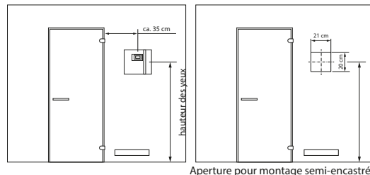
Aperture pour montage semi-encastré
