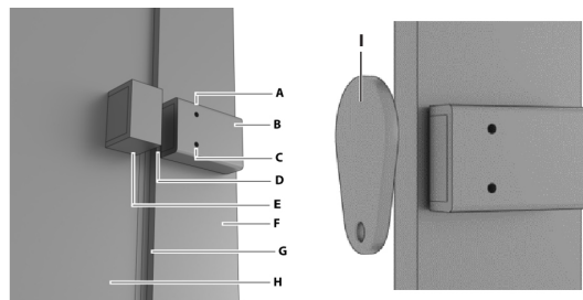
A. LED vihreä B. RFID yksikkö C. LED punainen D. Oviväli E. Ovimagneetti F. Ovikehys G. Oven välyys H. Ovilasi I. RFID-tunniste
