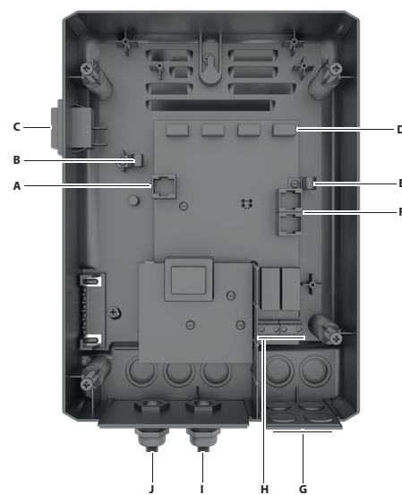
A. RFID-yksikön liitin B. Kaapelin vedonpoisto C. Päävirtakytkin D. Valoverhon liitin E. Kaapelin vedonpoisto F. Väyläyhteyden liitin G. Kaapeliläpivienni valoverholle H. Liitin turvapiirille (STB) I. Kaapeliläpivienni - virtalähteen liitântä J. Kaapeliläpivienni - ohjauskeskuksen liitântä
